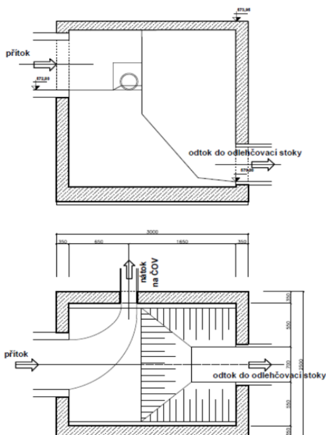
ODLEHČOVACÍ KOMORA stoka "A" před ČOV I.
